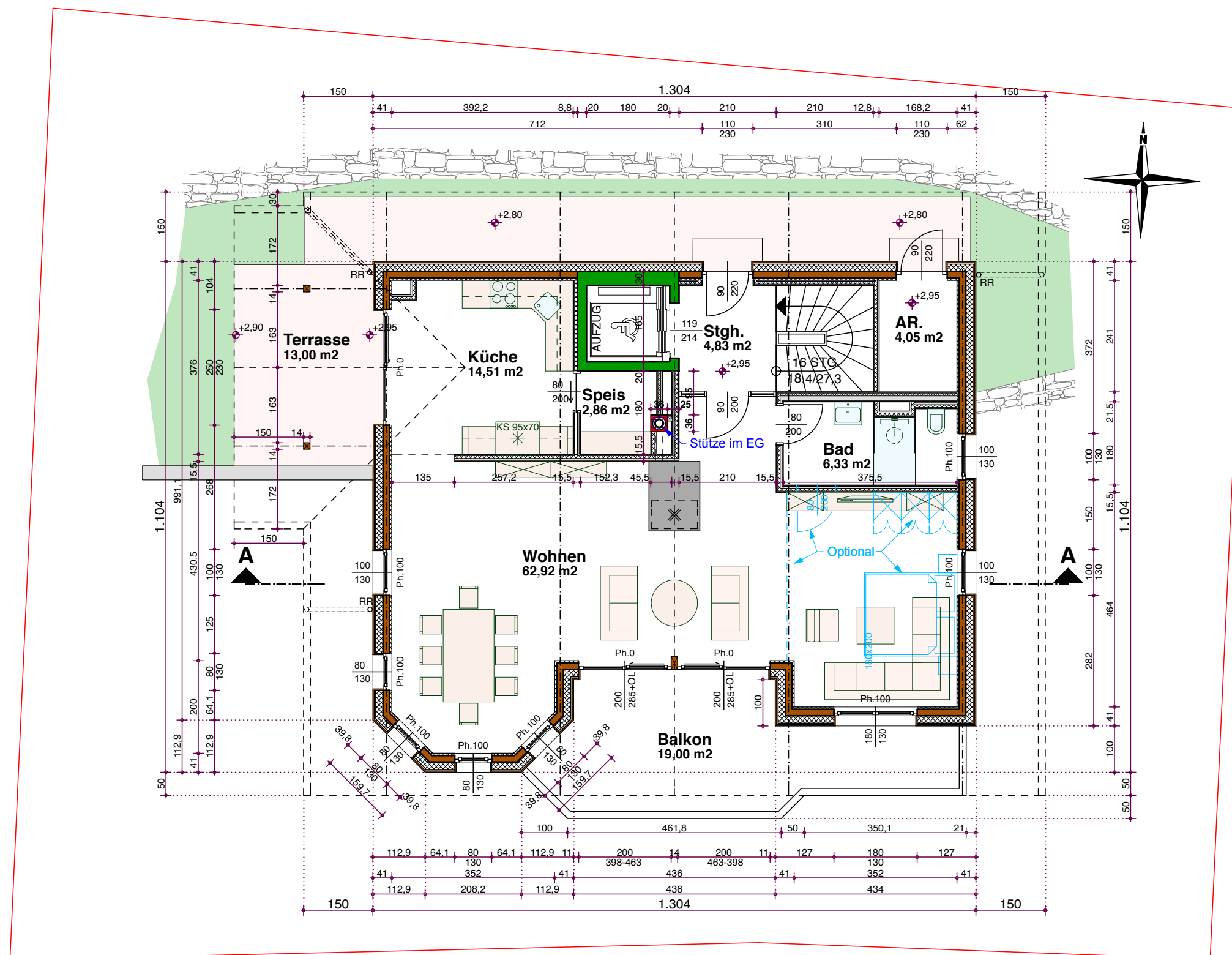
Obergeschoss
