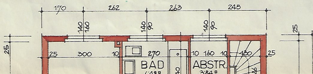
OBERGESCHOSS
