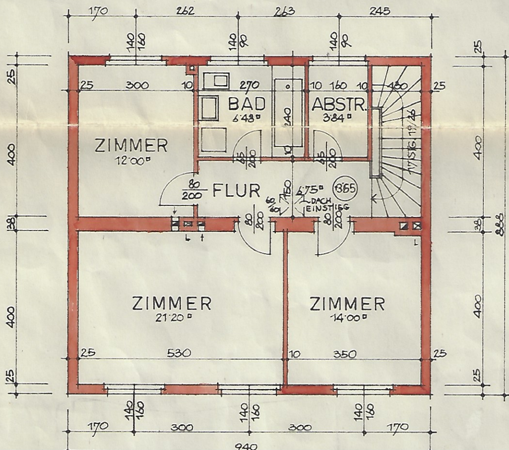
OBERGESCHOSS
