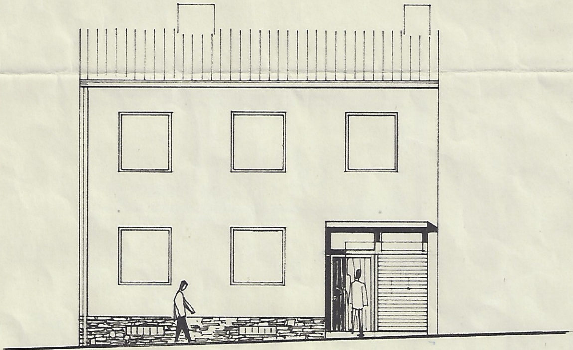
STRASSENANSICHT
